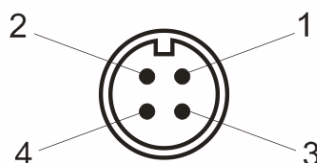
Рисунок 3.7 Разъем подключения преобразователей 1 – сигнал “А” линии RS-485 3 – общий провод 2 – сигнал “В” линии RS-485 4 – питание +12 В
